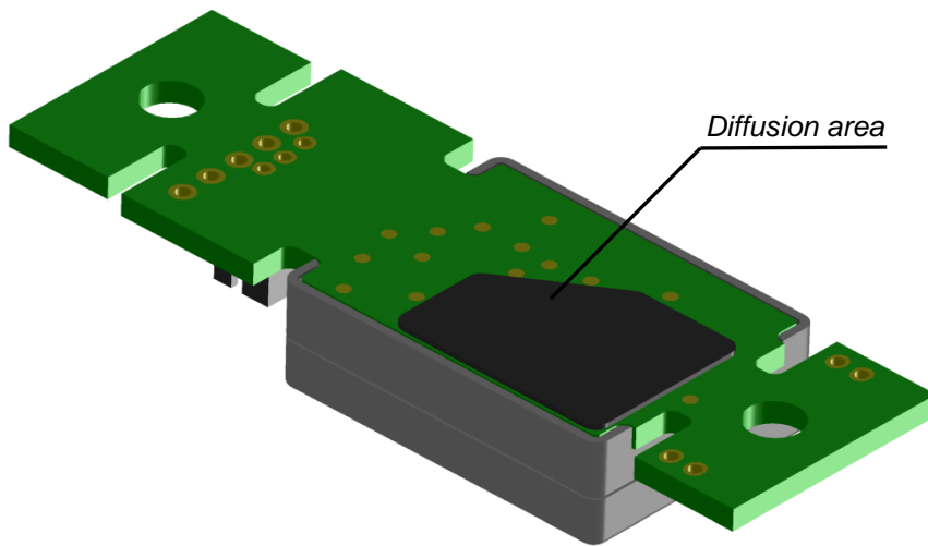
Figure 4. Gas diffusion area SenseAir ® S8-4B
